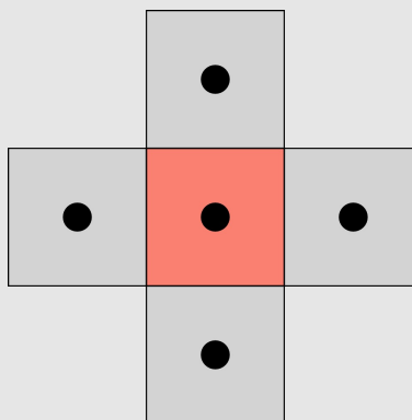
4-connectité
