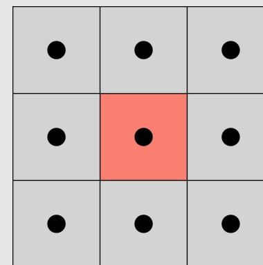
8-connectité
